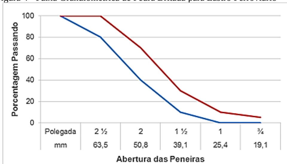
Figura 4 - Faixa Granulométrica de Pedra Britada para Lastro Ferroviário
