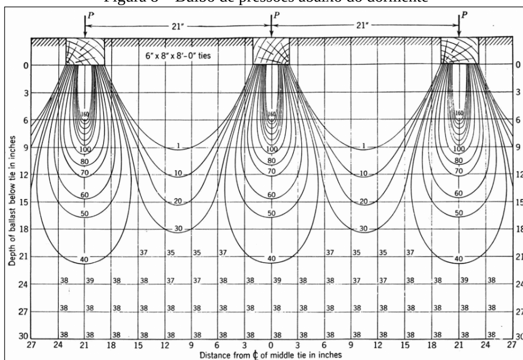
Figura 8 – Bulbo de pressões abaixo do dormente
