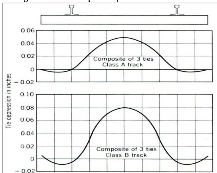
Figura 6 - Distribuição das pressões sob os dormentes
