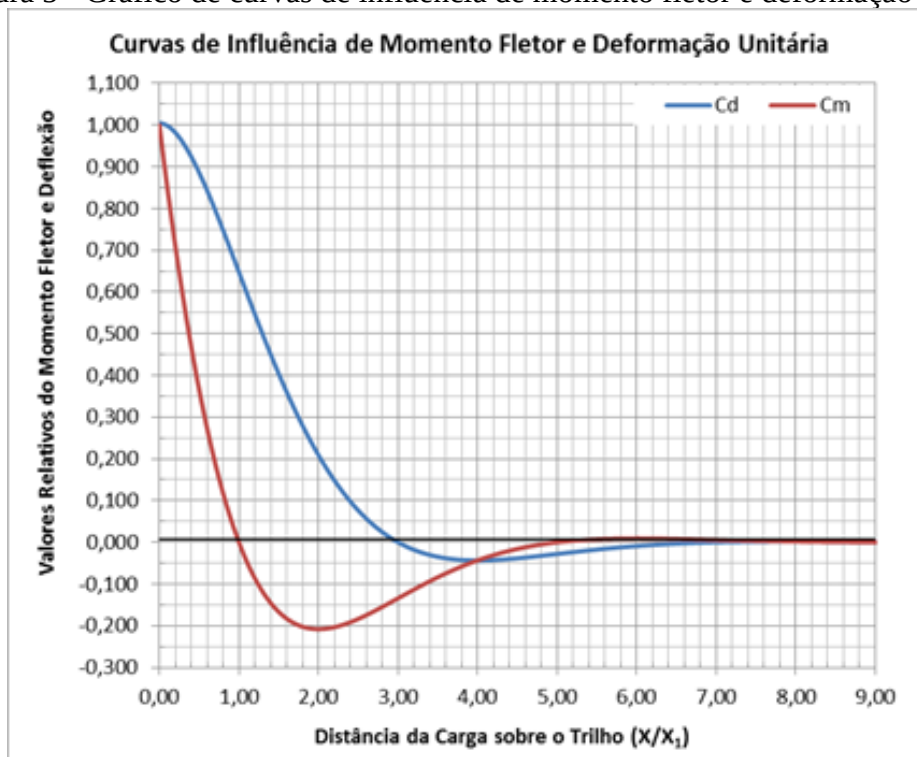
Figura 5 - Gráfico de curvas de influência de momento fletor e deformação unitária
