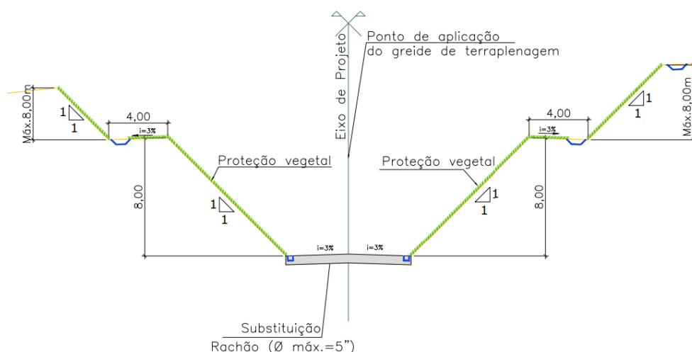
Figura 2 – Substituição para cortes em 1ª Categoria – CBR < 3\% .
